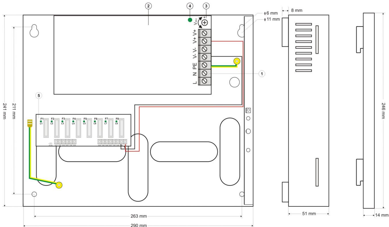
Rys.3. Widok zasilacza.
